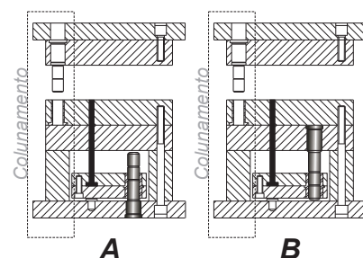
Opções de Montagem - M3
