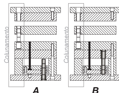
Opções de Montagem - M6
